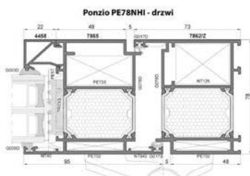
Przekrój drzwi Optimum HI
